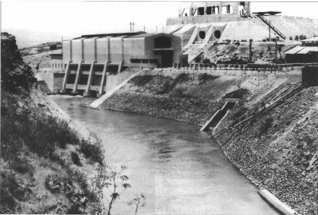
Usina hidroeléctrica en Naharaim, programada por el Ing. Piniás Rutenberg. Archivo fotográfico - KKL.
